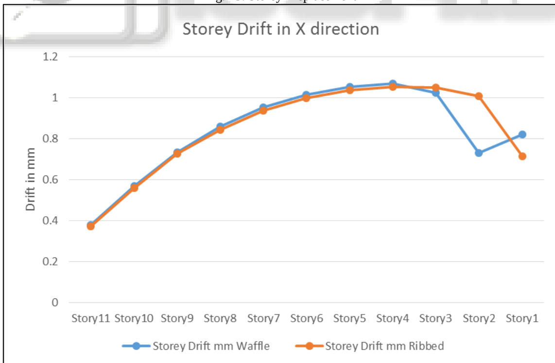
Fig. 14: Storey Drift
