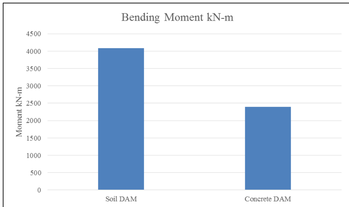
Fig. 10: Bending Moment
