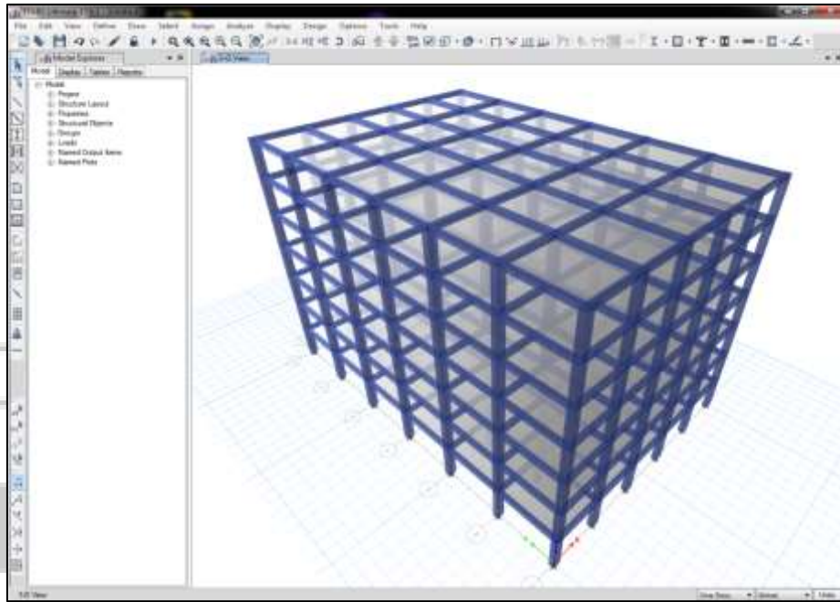
Fig. 6: Bare Frame
