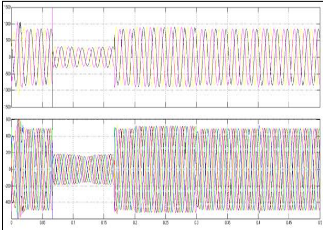
Fig. 4: Non Linear Load Output
