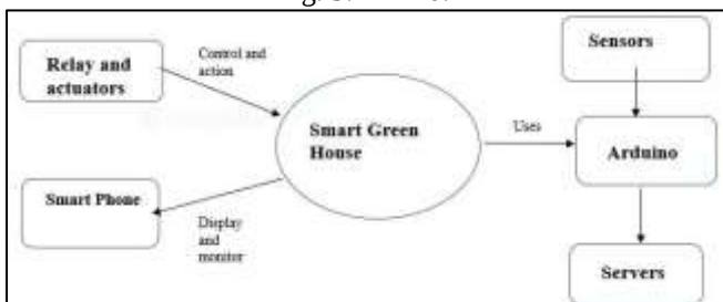
Fig. 4: DFD 1.
