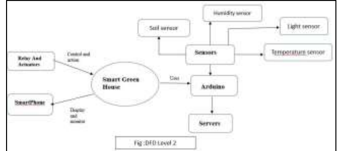
Fig. 5: DFD 2.
