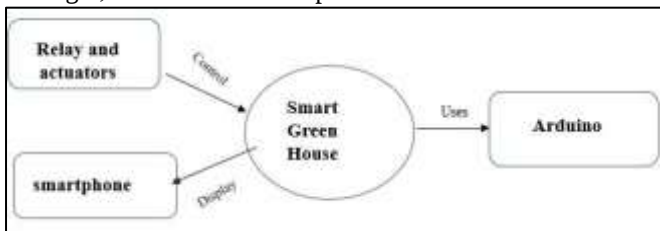
Fig. 3: DFD 0.
